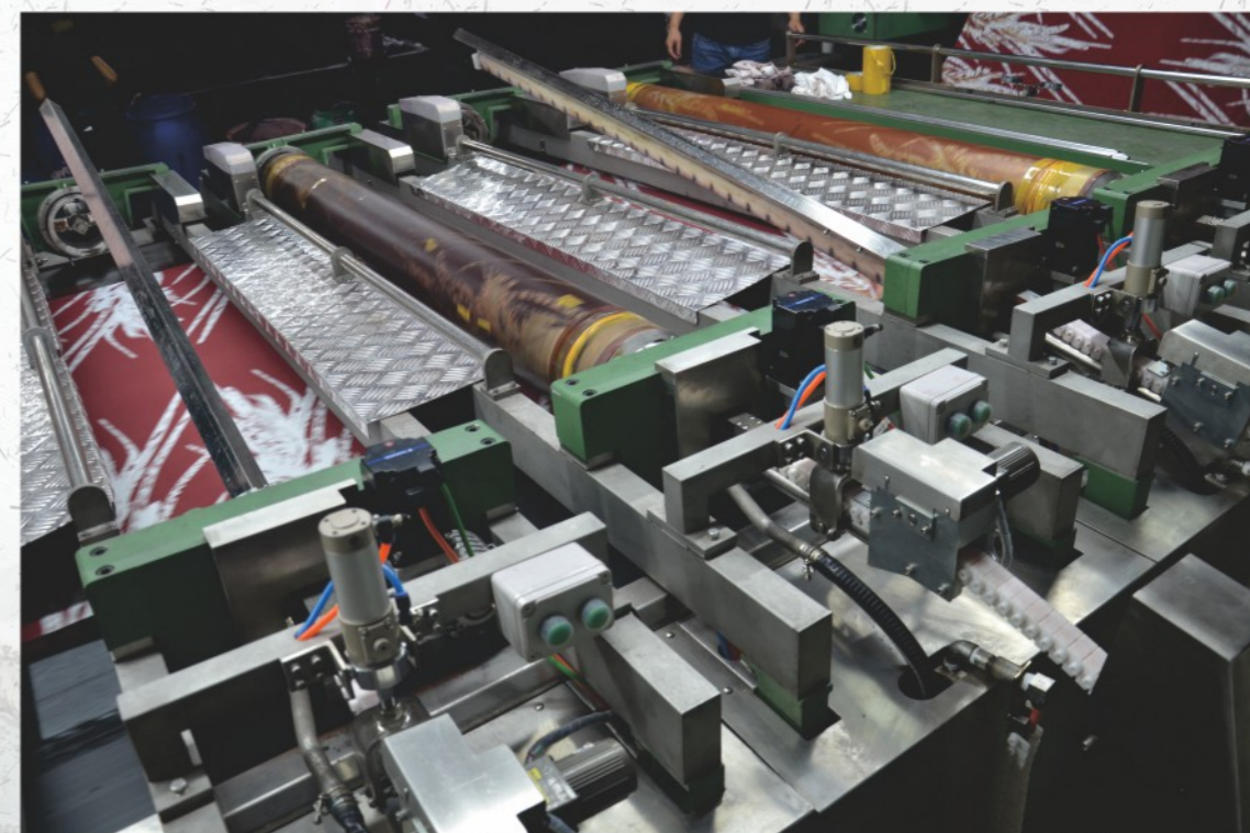
各印花单元及导带均采用伺服马达驱动，自动对花，印花速度快，印花精度高。 换色时不用拆卸、色管、磁棒、圆网、有效地保护了网筒的使用寿命。
